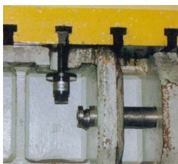
MC-Clamp, övre verktyg, ej fastspänt läge
